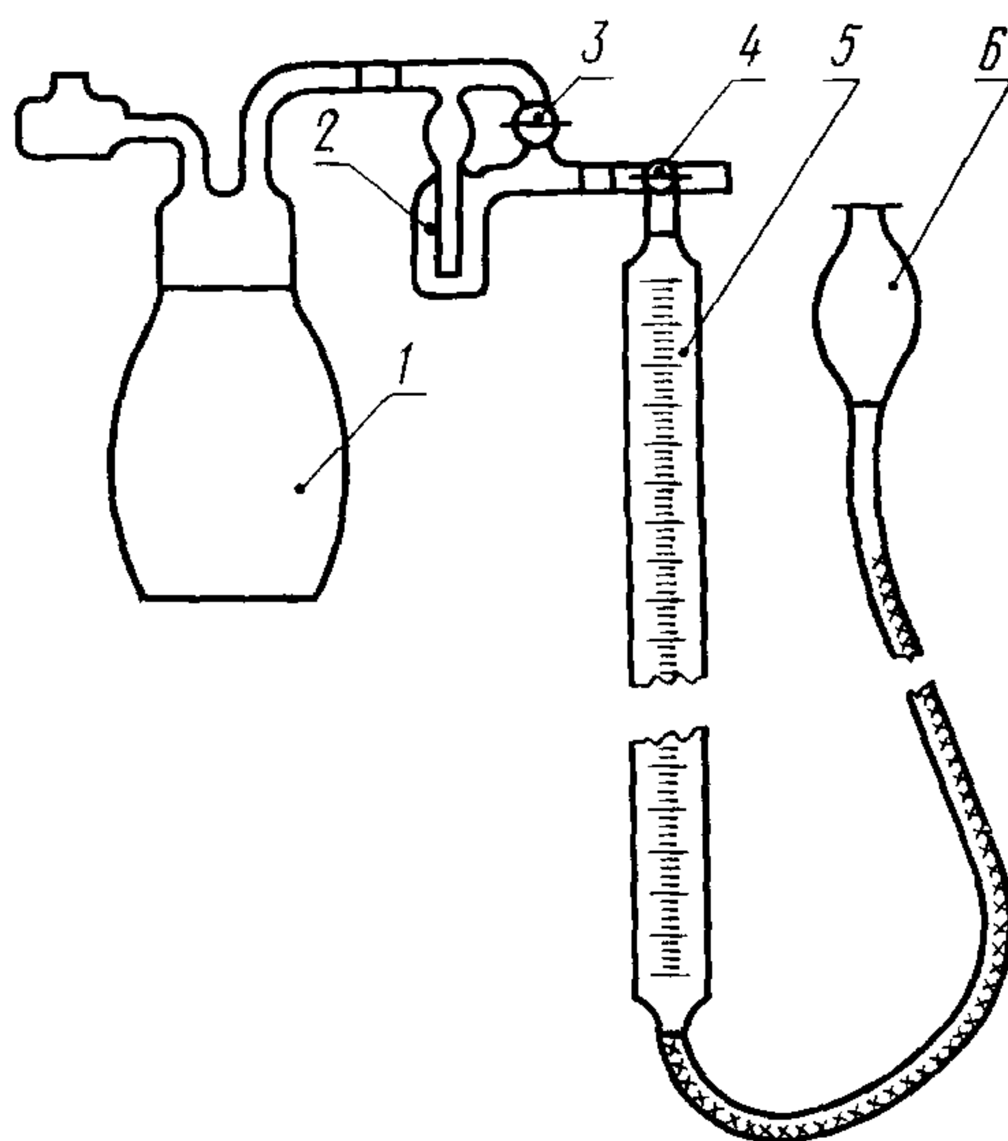
Прибор для определения массовой доли воды
